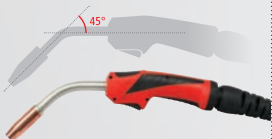
Torche de soudage manuelle MIG/MAG refroidie par gaz ou par eau
